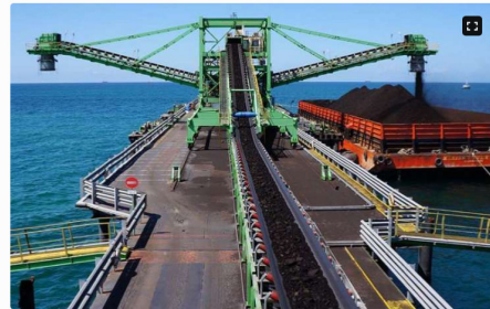
Proses pengapalan batu bara dari conveyor belt ke kapal tongkang. - atminvestasi.com
